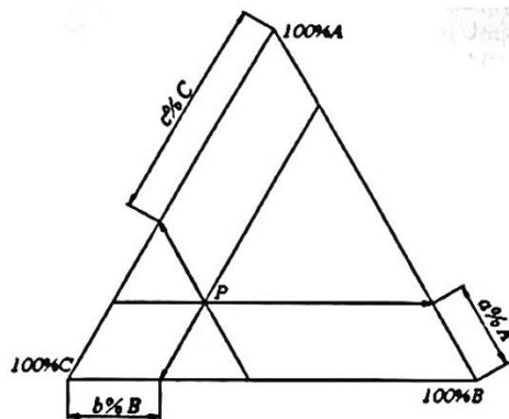
Rysunek 1. Skład układu trójskładnikowego.
