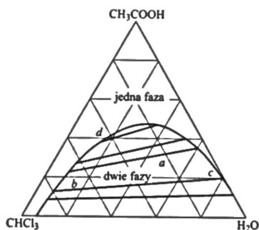
Rysunek 2. Ciekły układ kwas octowy - chloroform - woda pod ciśnieniem 1 bar w temp. 180°C.
