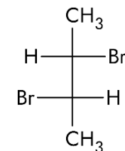
(2S,3S)-2,3-dibromobutan
