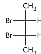
mezo-2,3-dibromobutan
