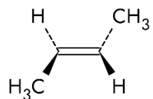
(2E)-but-2-en
