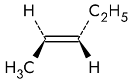
(2E)-pent-2-en
