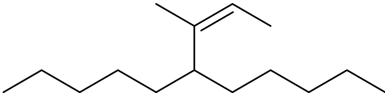
6-(but-2-en-2-yl)undekan
