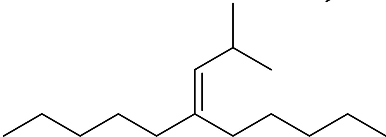
6-(2-metylopropylideno)undekan
