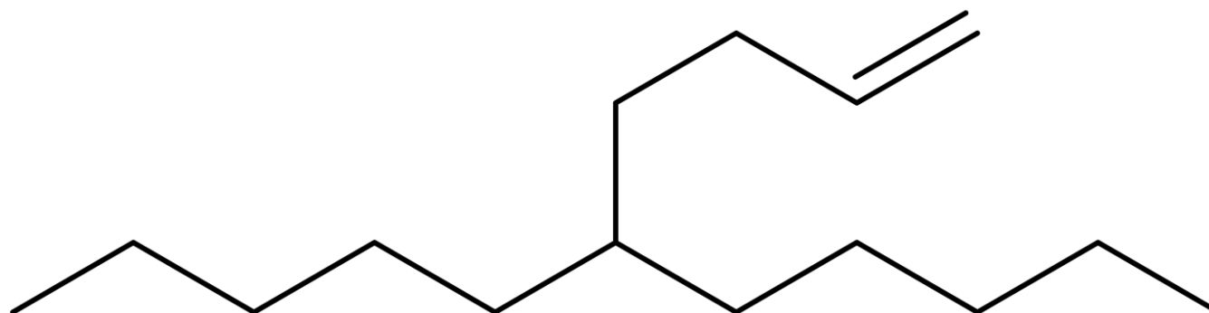
6-(but-3-en-1-yl)undekan
