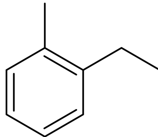
1-etylo-2-metylobenzen
