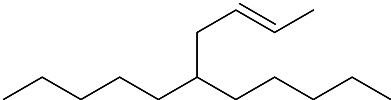
6-(but-2-en-1-ylo)undekan
