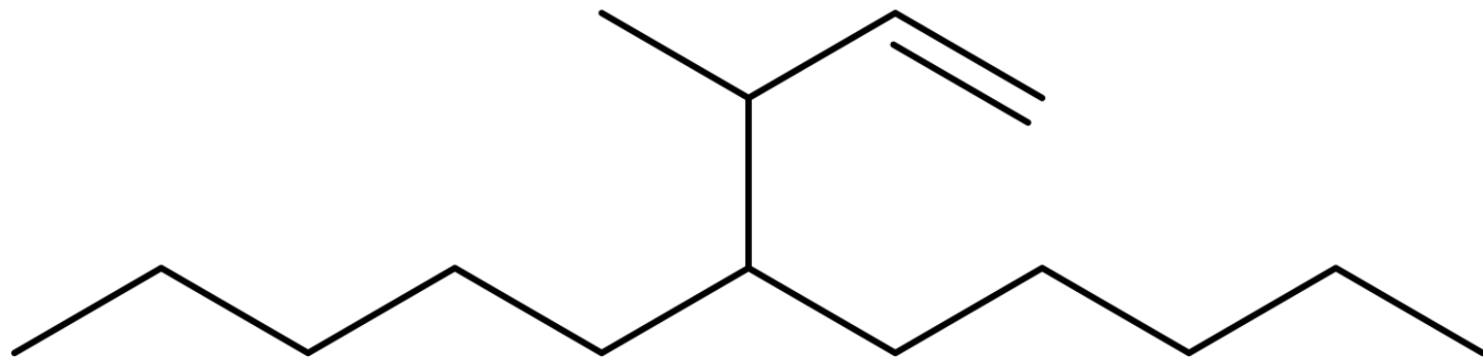
6-(but-3-en-2-yl)undekan
