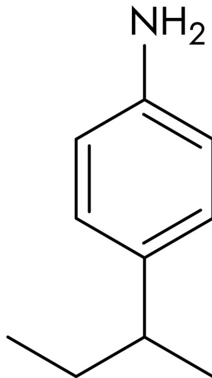
4-(but-2-ylo)anilina
