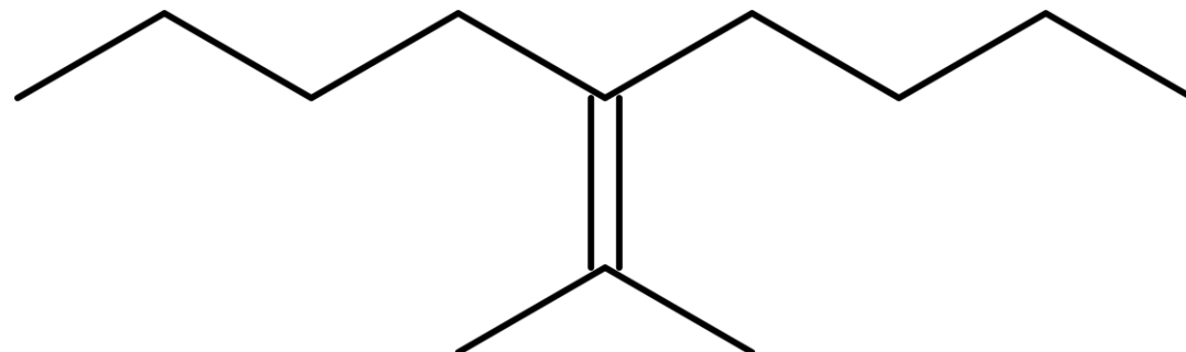
5-(propan-2-ylideno)nonan
