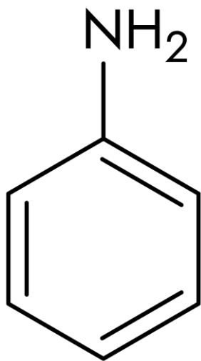
anilina
