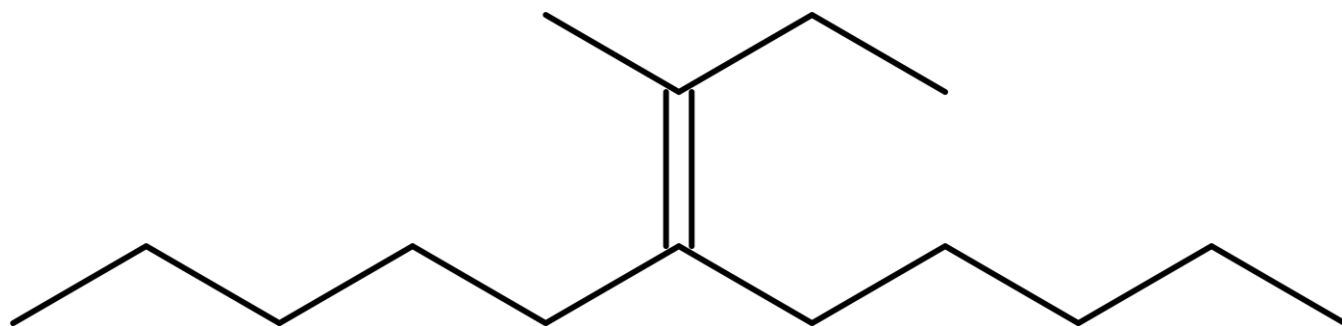
6-(but-2-ylideno)undekan
