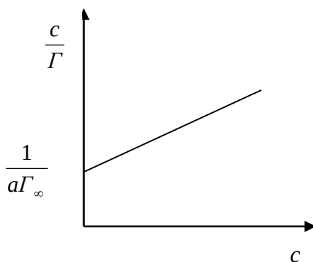
Rys. 5. Wykres zależności c/\Gamma od stężenia substancji powierzchniowo czynnej.
