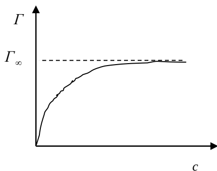
Rys. 4. Zależność nadwyżki powierzchniowej \Gamma od stężenia surfaktanta w roztworze.
