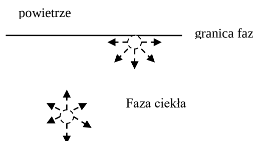
Rys. 1. Oddziaływanie międzycząsteczkowe w głębi fazy ciekłej i na granicy faz powietrze – faza ciekła.
