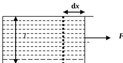
Rys. 1. Obliczanie pracy powierzchniowej.
