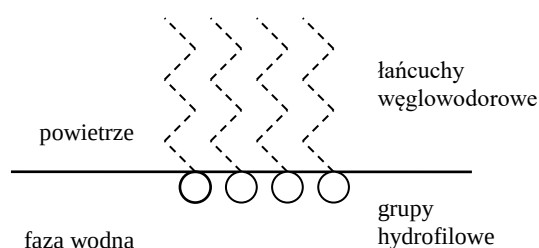
Rys. 2. Orientacja cząsteczek związków powierzchniowo aktywnych na granicy faz roztwór wodny – powietrze.
